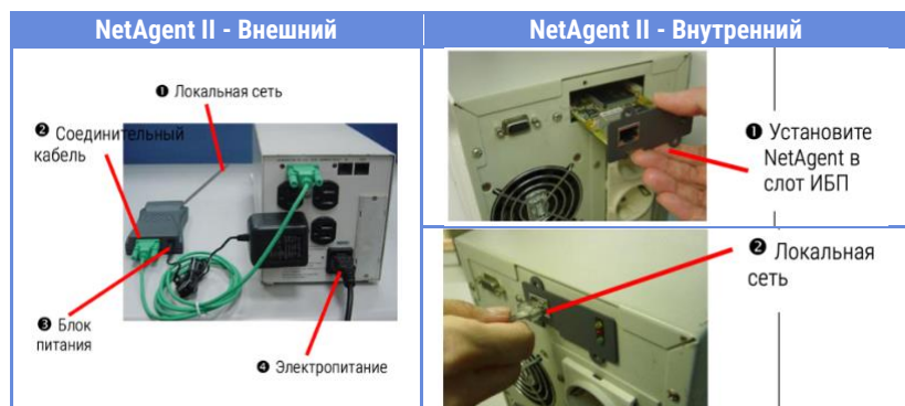
Рис.5. Установка NetAgent II
