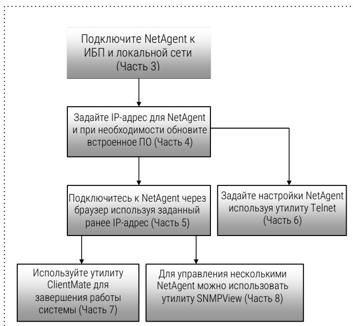
Рис.4. Блок схема установки NetAgent
