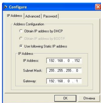
Рис.8 Конфигурирование Netility
