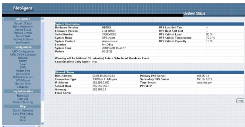
Рис.16 трехпортовый NetAgent ИБП
