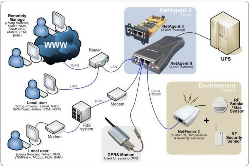
Рис.2. 3-портовый NetAgent II схема подключения
